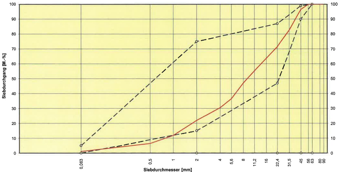
Sieblinienbereiche NGK 0/45 FSS nach TL SoB-StB
